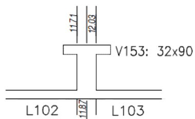
DETALLE VIGA-LOSA
